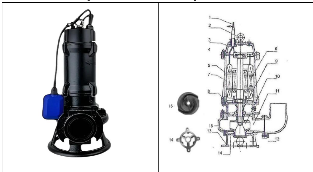
Figura 06 - Bomba modelo Lepono WQ25-15-22
