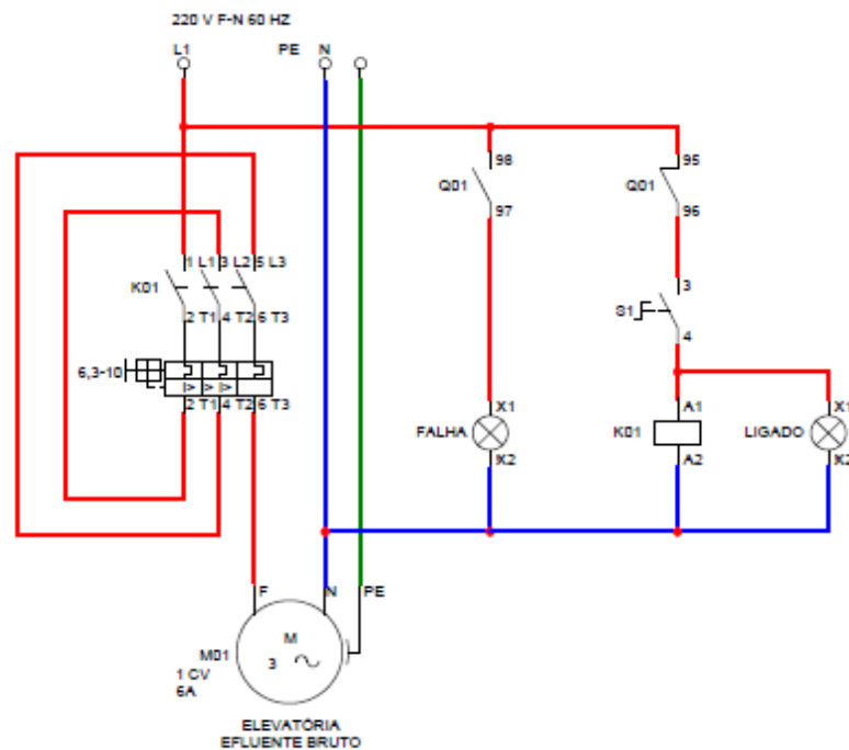
Figura 10 – Diagrama Elétrico modelo LSWm100CA (1,0 CV).
