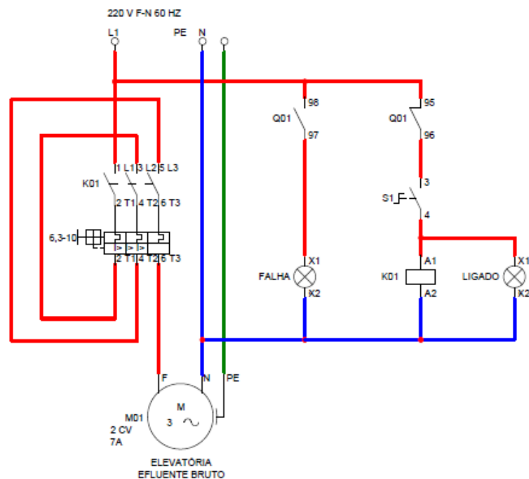
Figura 11 – Diagrama Elétrico modelo LSWm200CA (2,0 CV).
