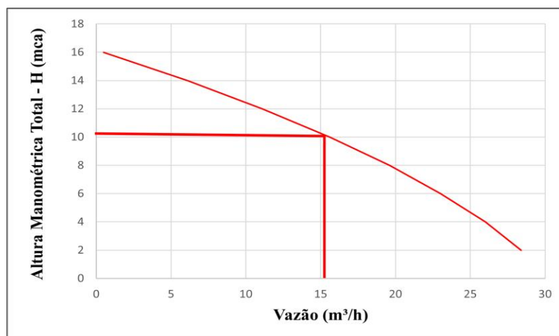
Figura 08 – Exemplo da curva característica da bomba LSWm200CA de 2 CV.
